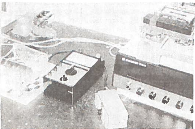
Apparatuur "Omega". Zender: 5-traps torrenbak met BLY87 in eindtrap. Ant.: 4-elements.
