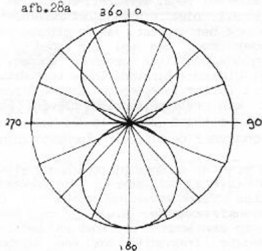
afb. 28: Een eenvoudige Raamantenne.
