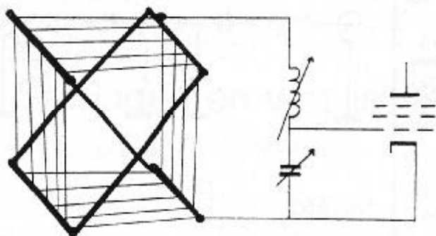
RAAMANTENNE
