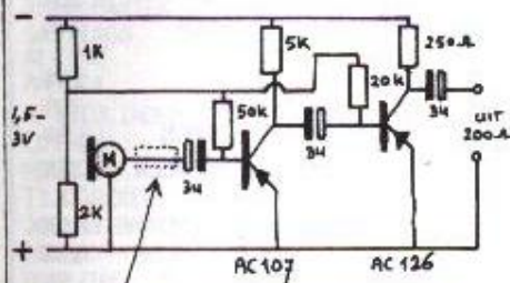
MIKE-VERSTERKER
